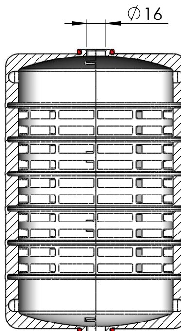
SECCIÓN A-A
